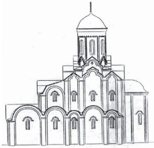
Рэканструкцыя Спаскай царквы ў Полацку, паводле даследаванняў 2015 г. Аўтар - П. Зыкаў.
